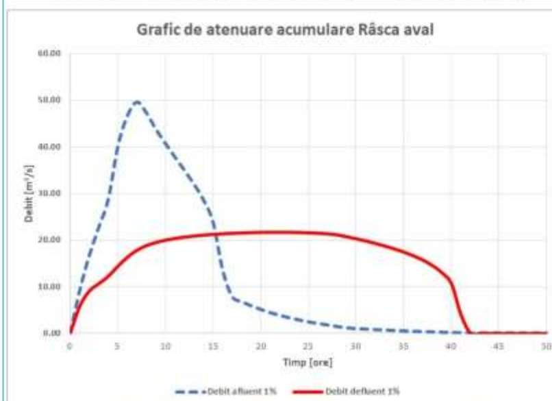
Figura 4-3: Grafic de atenuare pentru acumularea Râsca aval în scenariul Q1%
