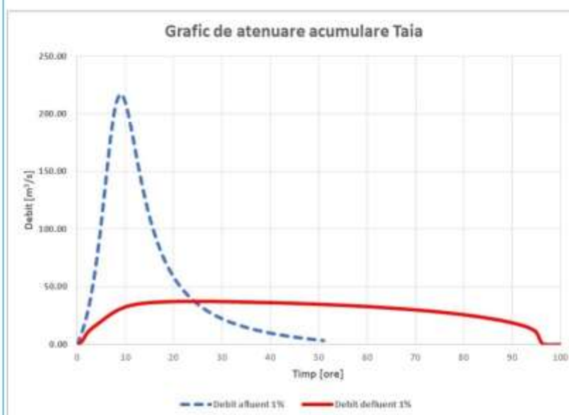
Figura 4-4: Grafic de atenuare pentru acumularea Taia în scenariul Q1%
