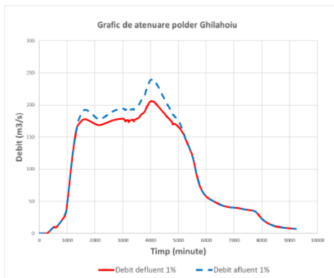
Figura 4-4 – Graficul de atenuare pentru polderul Ghilahoiiu la 1%
