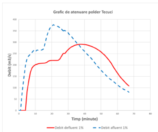
Figura 4-10 – Graficul de atenuare pentru polderul Tecuci la 1%
