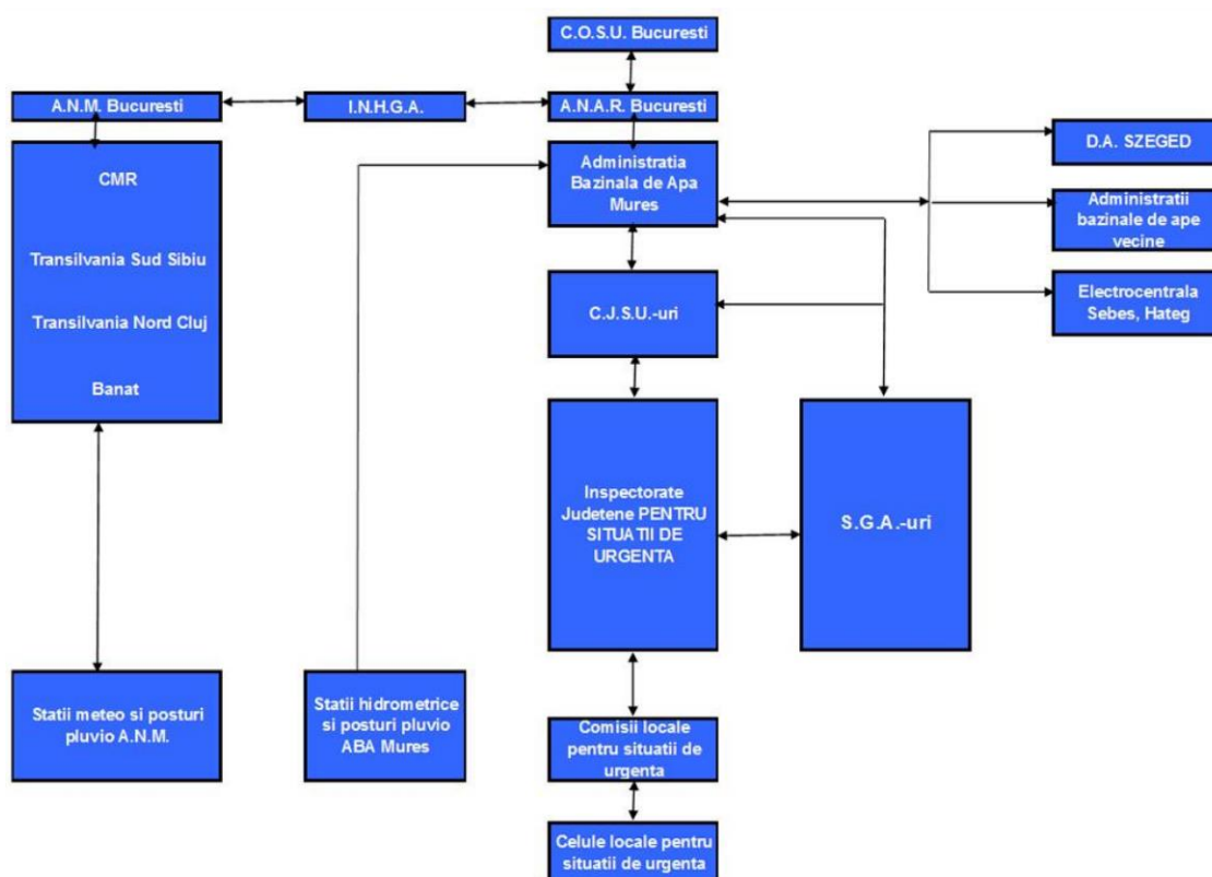
Figura 3.7.1 Schema de gospodărire a apelor existentă în bazinul hidrografic Mureș
